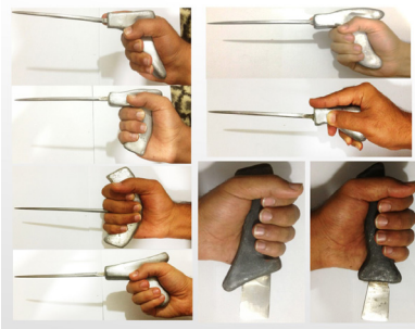
ابزارهای بازطراحی‌شده کفی‌سازی گیوه
