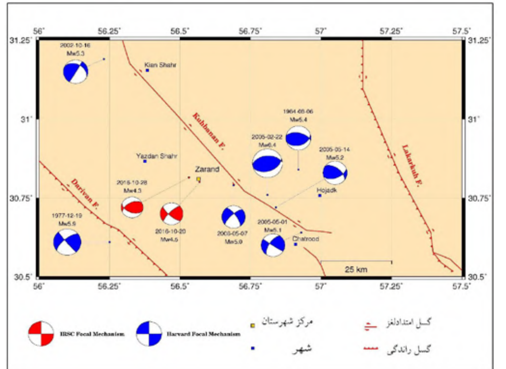
شکل ۴: سازوکار کانونی زمین‌لرزه‌های بزرگ‌تر از ۴ ثبت‌شده در اطراف شهر زرنند بدون حساب زمین‌لرزه عصر گذشته مکانیسم دو زمین‌لرزه اخیر با رنگ قرمز مشخص شده است.
