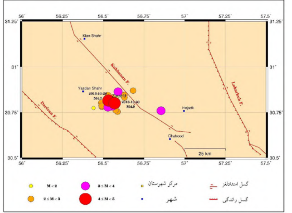
شکل ۱: توزیع مکانی رومرکز زمین‌لرزه‌های اخیر زرنند کرمان ۱۳۹۵ / ۷ / ۲۹ الی ۱۳۹۵ / ۸ / ۱۰
