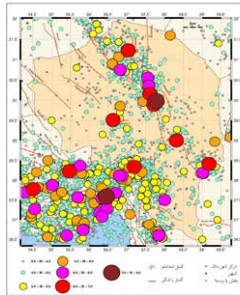
شکل ۲: زمین‌لرزه‌های تاریخی استان کرمان پیش از سال ۱۹۰۰ میلادی
